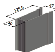
Perfil guía
